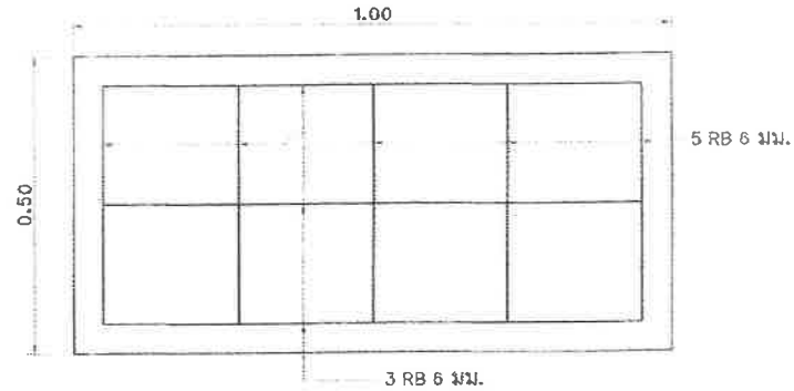
แบบขยายแปลนแผ่นพื้นรองท่อ คสล. มาตรฐาน 1 : 10
