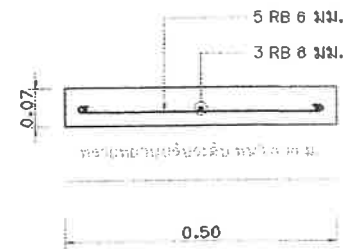
แบบขยายรูปตัดแผ่นพื้นรองท่อ คสล. มาตรฐาน 1 : 10
