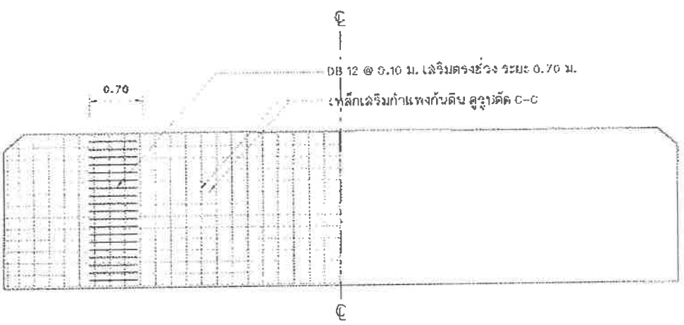
แบบขยายกำแพงกันดิน มาตราส่วน 1:50
