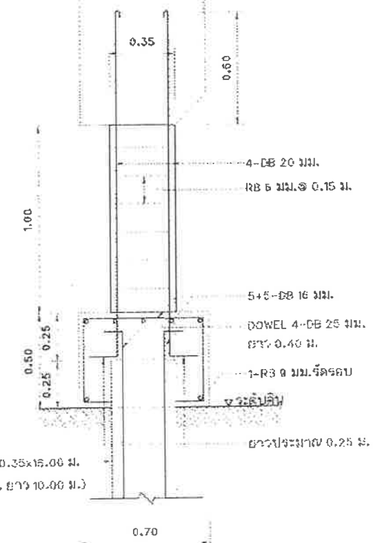
รูปตัดเสา C1 มาตรฐาน 1:20
