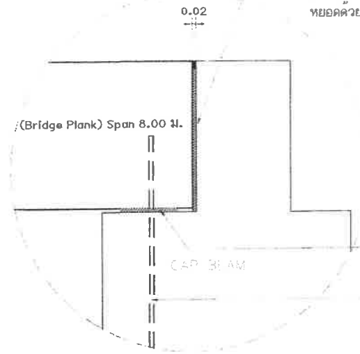
แบบขยาย CAP BEAM มาตราส่วน 1:10
