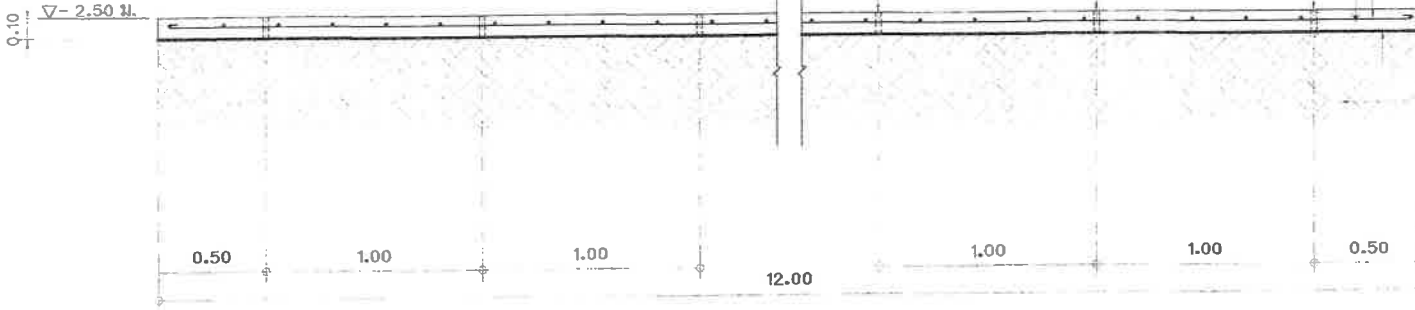
รูปตัดดาดท้องคลอง (สะพานที่ 2) มาตรฐาน 1:25
