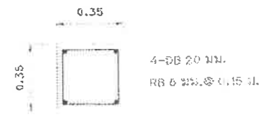
แบบขยายเสา C1 มาตรฐาน 1:20
