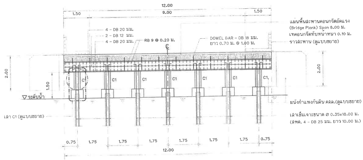
รูปตัดโครงสร้าง A - A (สะพานที่ 2) มาตราส่วน 1:75
