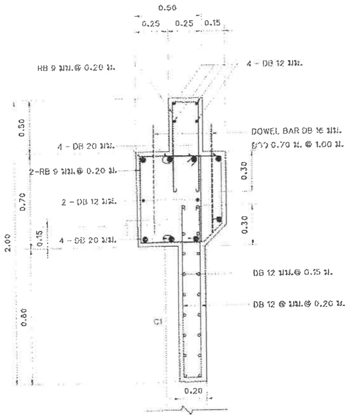
รูปตัดโครงสร้าง B - B (สะพานที่ 1) มาตรฐาน 1:20
