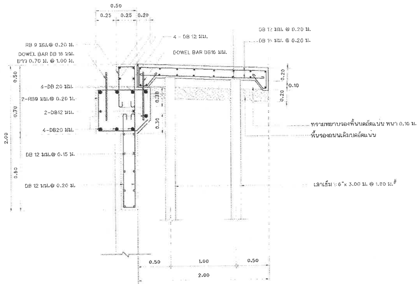
รูปตัดการเชื่อมสะพาน และคิวงถนน คสล. (ฝั่งถนนล้ามีคคิ)
