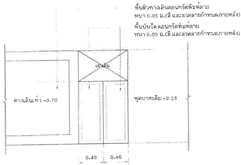
แบบขยายรูปตัดบันได ST2 มาตราส่วน 1:25
