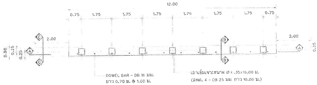
ขยายโครงสร้างสะพาน (สะพานที่ 1) มาตราส่วน 1:75
