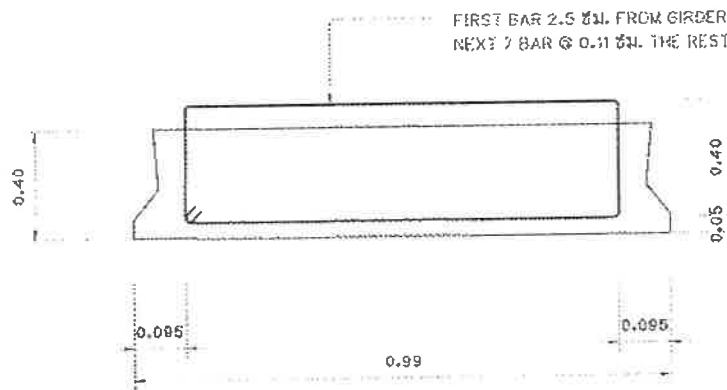
PLANK 11.00 M. SPAN
