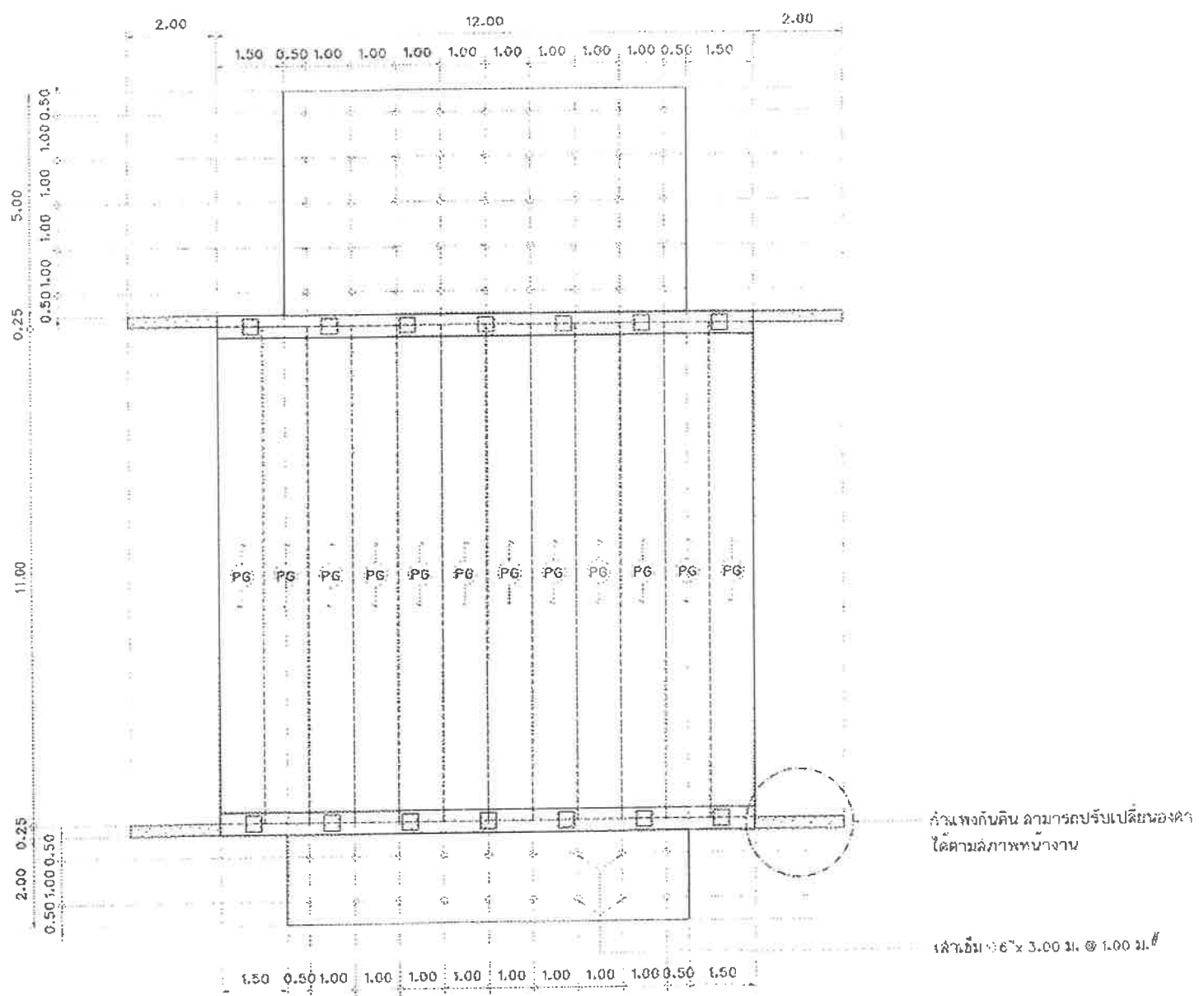
แปลนโครงสร้างสะพาน คสล. (สะพานที่ 1) มาตราส่วน 1:100
