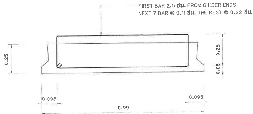
PLANK 8.00 ม. SPAN
