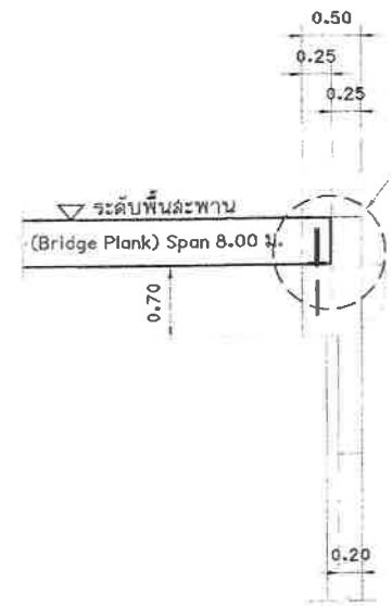
CAP BEAM มาตราส่วน 1:50
