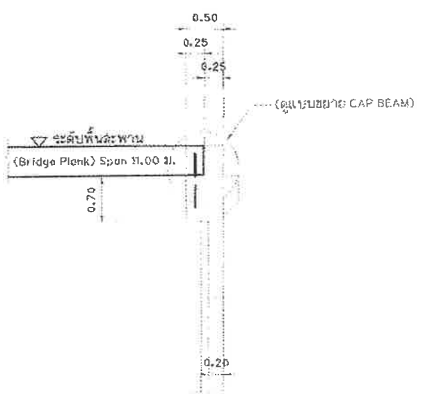
CAP BEAM มาตราส่วน 1:50
