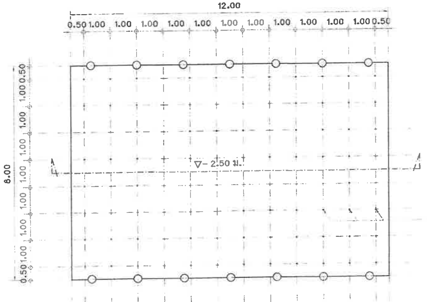
แปลนเสาเข็มดาดท้องคลอง (สะพานที่ 2) มาตรฐาน 1:100
