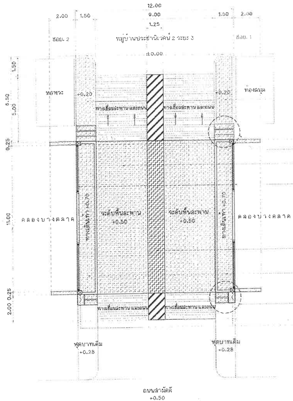
แปลนสะพาน คสล. (สะพานที่ 1) มาตราส่วน 1 : 125
