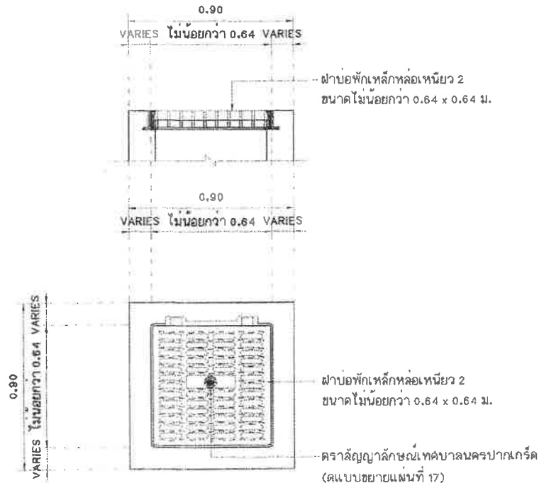
แบบขยายฝาครอบเหล็กหล่อเหนียว 2
