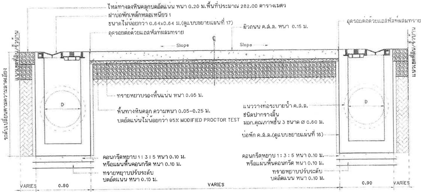
แบบขยายรูปตัด 2 (แบบมีไหลทางลงหินคลุก)
