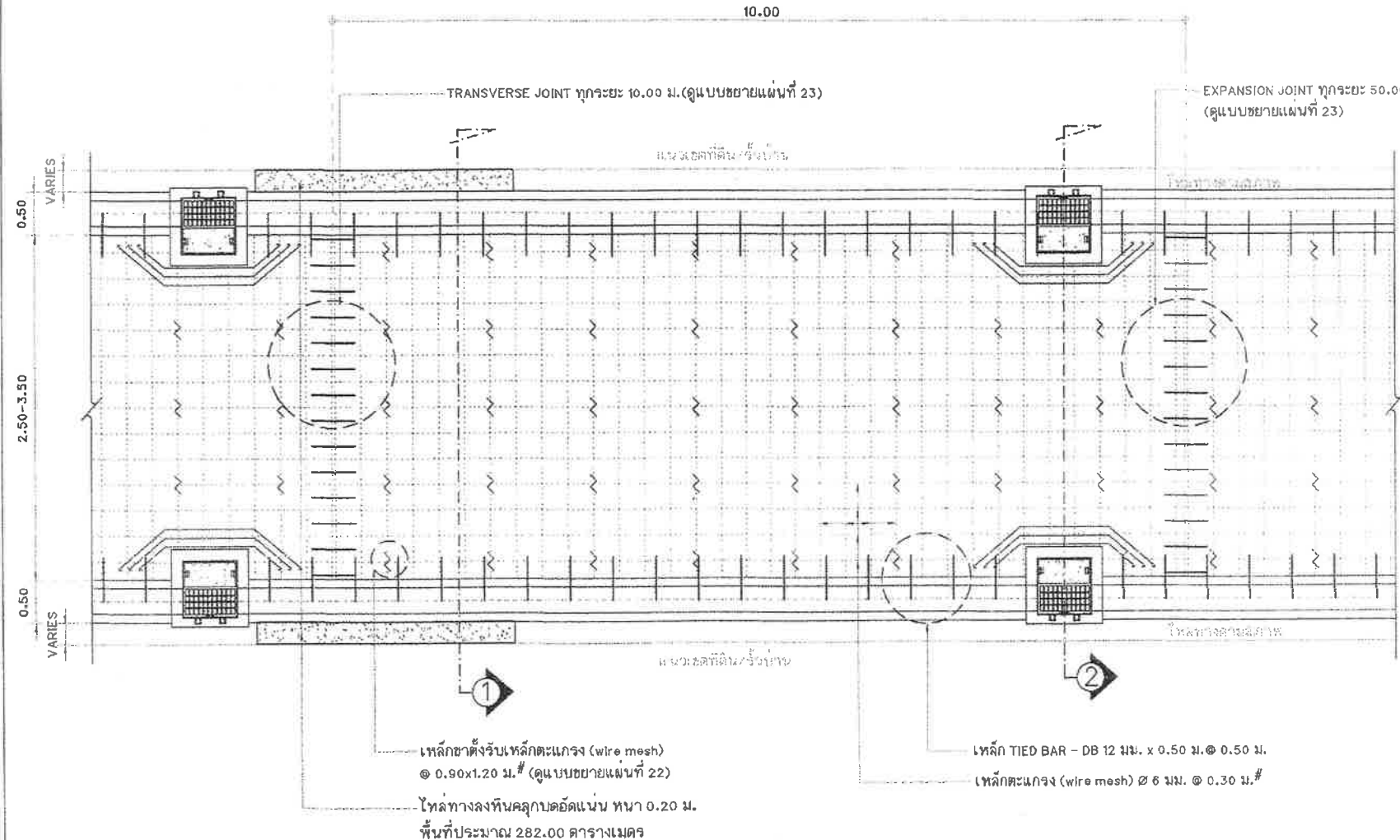
แปลนการวางเหล็กตะแกรงและรอยต่อถนน คสล. (แบบมีโหลทางลงหินคลุก) มาตรฐาน 1 : 50
