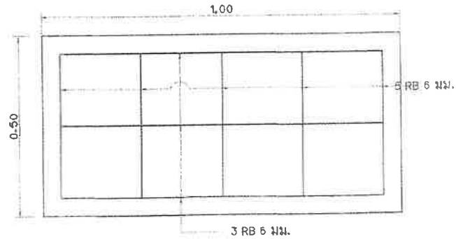
แบบขยายแปลนพื้นร่องท่อ มาตรฐาน 1 : 10
