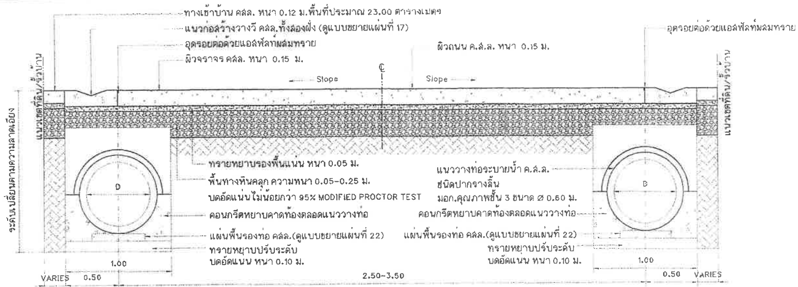
แบบขยายรูปตัด 1 (แบบมีทางเข้าบ้าน คสล.)
