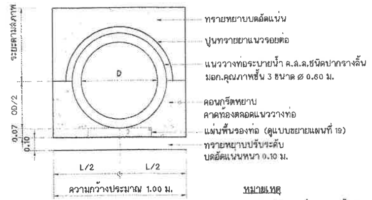
แบบขยายการวางท่อระบายน้ำ คสล. มาตราส่วน 1:20
