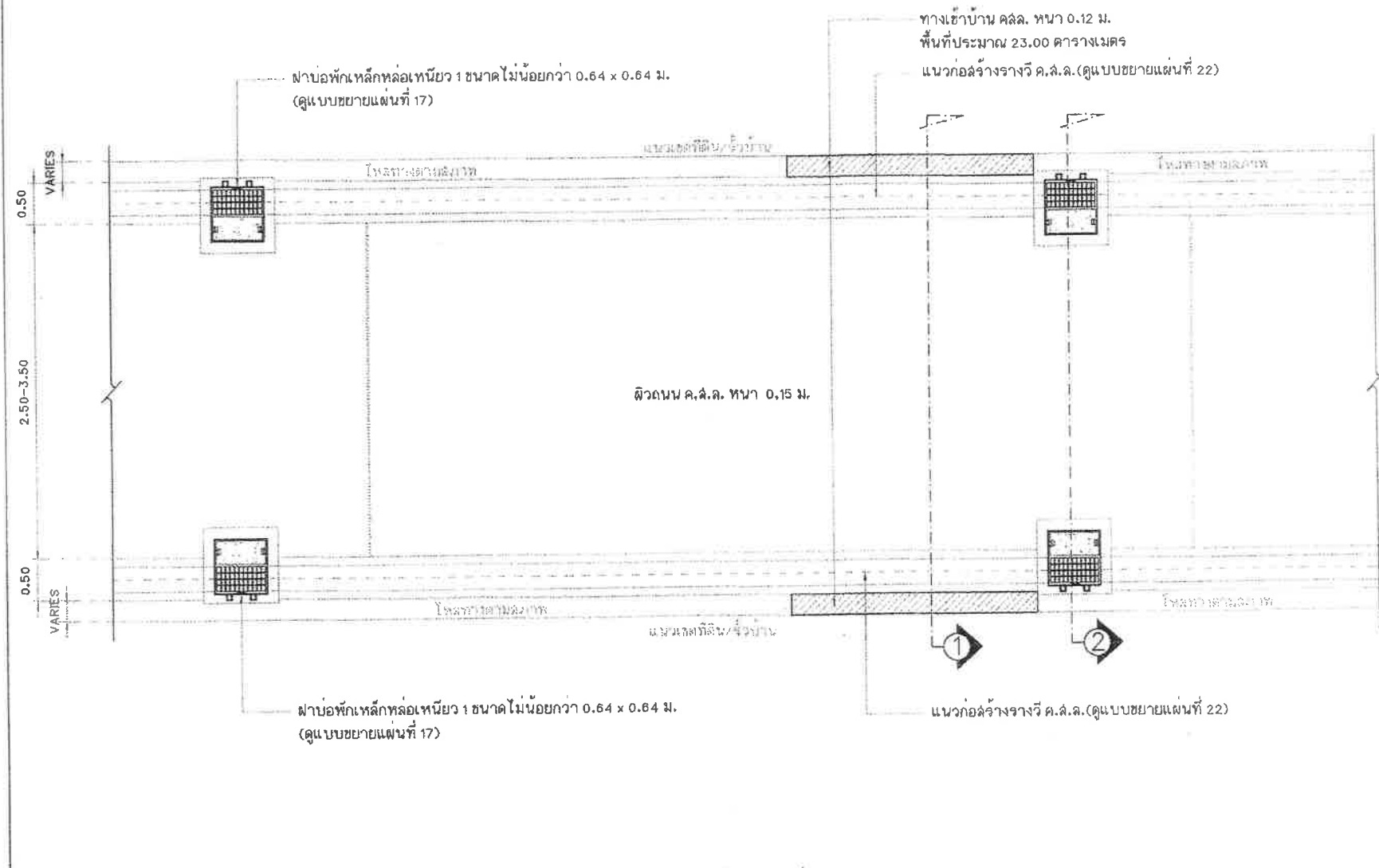
แปลนถนน และการวางบ่อพัก คสล. (แบบมีทางเข้าบ้าน คสล.) มาตราส่วน 1 : 50
