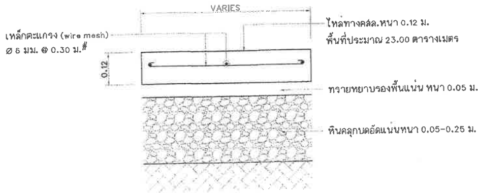
แบบขยายรูปตัดทางเข้าบ้าน คสล.หนา 0.12 ม. มาตรฐาน 1 : 10
