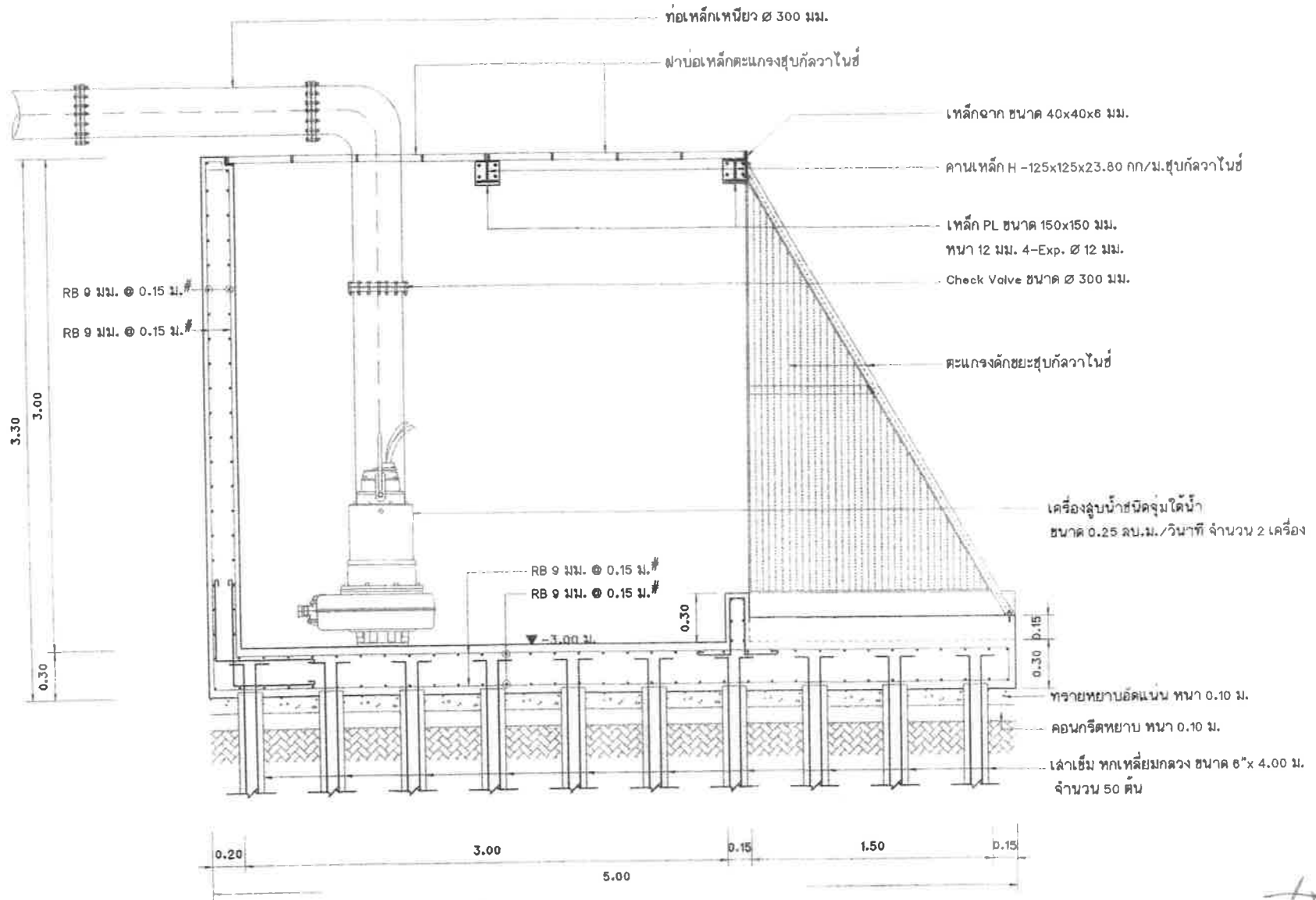
รูปตัด โครงสร้าง ๑ บ่อสูบน้ำ คลล. มาตราส่วน 1:25
