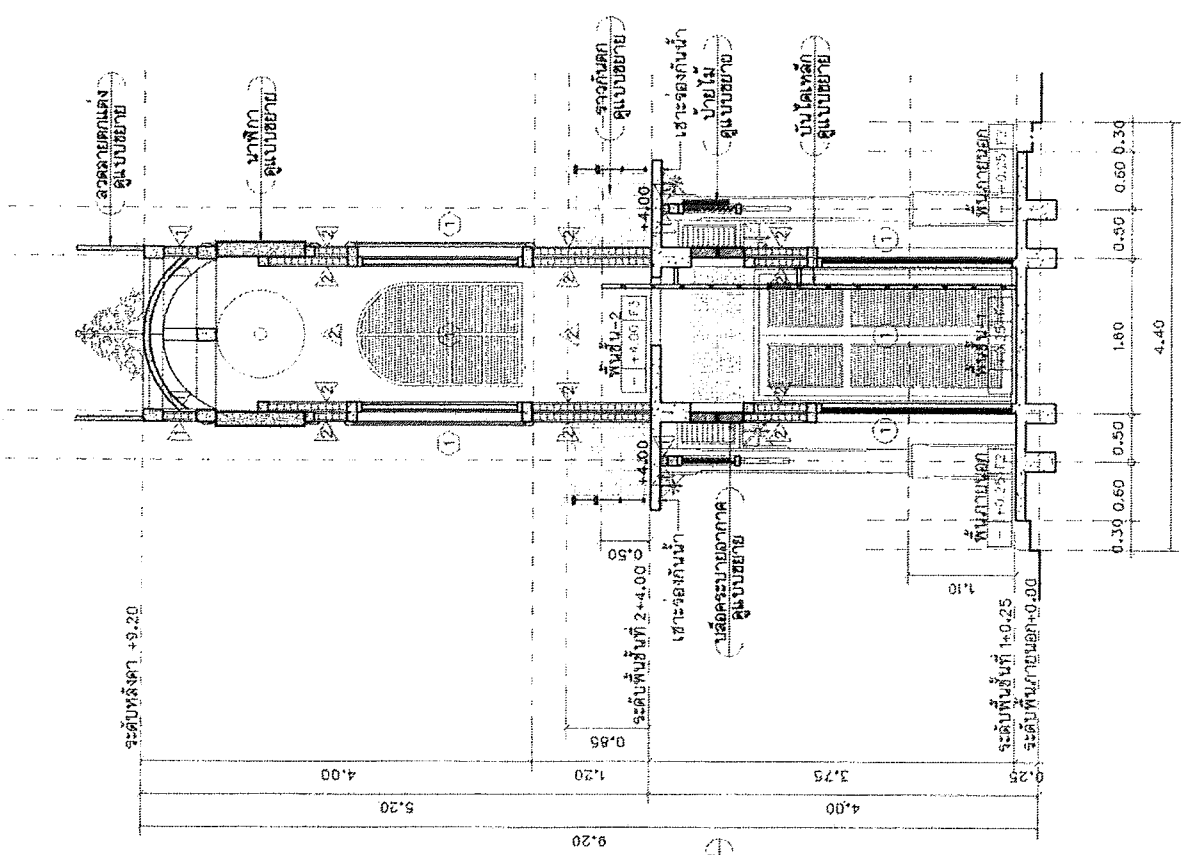
รูปตัด-B SCALE 1:50
