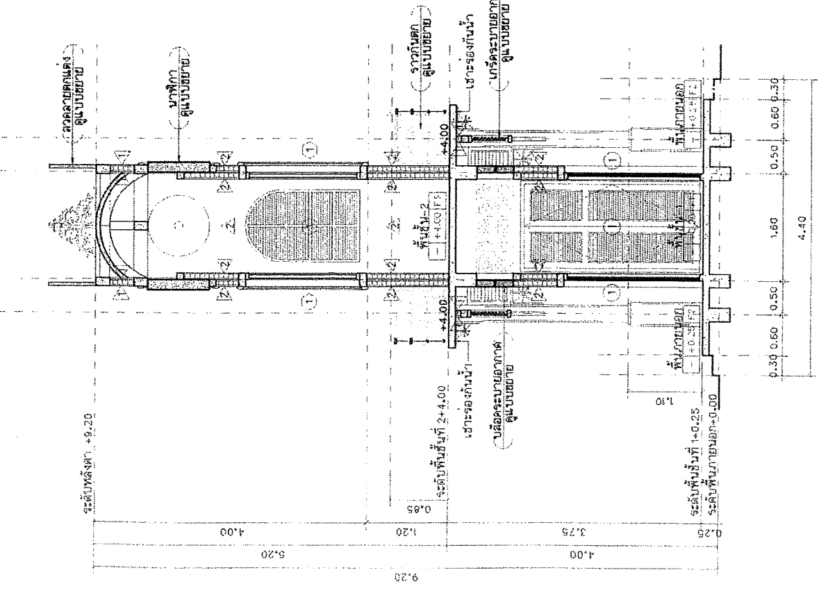
รูปตัด-A SCALE 1:50
