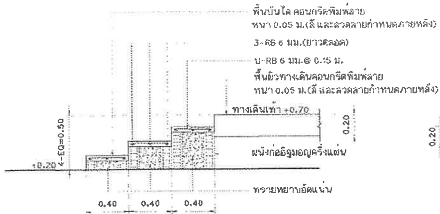
แบบขยายรูปตัดบ้นไค ST1 มาตราส่วน 1: 25
