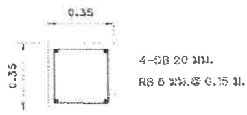
แบบขยายเสา C1 มาตราส่วน 1:20
