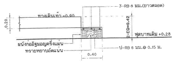
แบบขยายรูปตัดบันได ST2 มาตราส่วน 1:25
