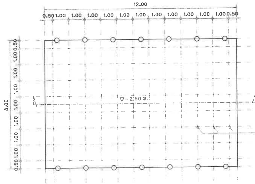
แปลนเล้าเชื่อมดาดท้องคลอง (สะพานที่ 2) มาตรฐาน 1:100
