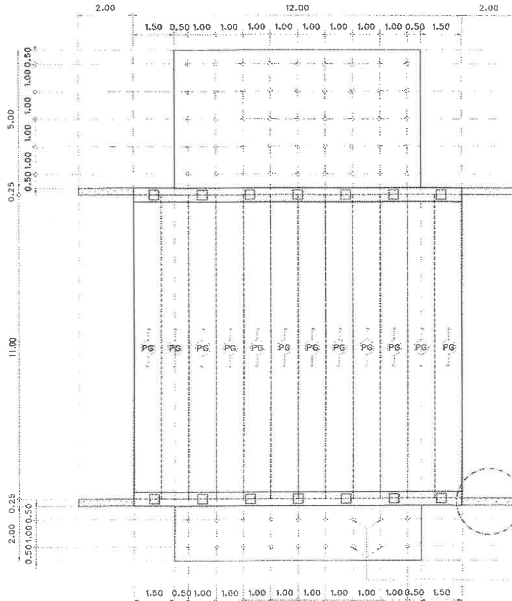
แปลนโครงสร้างสะพาน คสล. (สะพานที่ 1) มาตรฐาน
