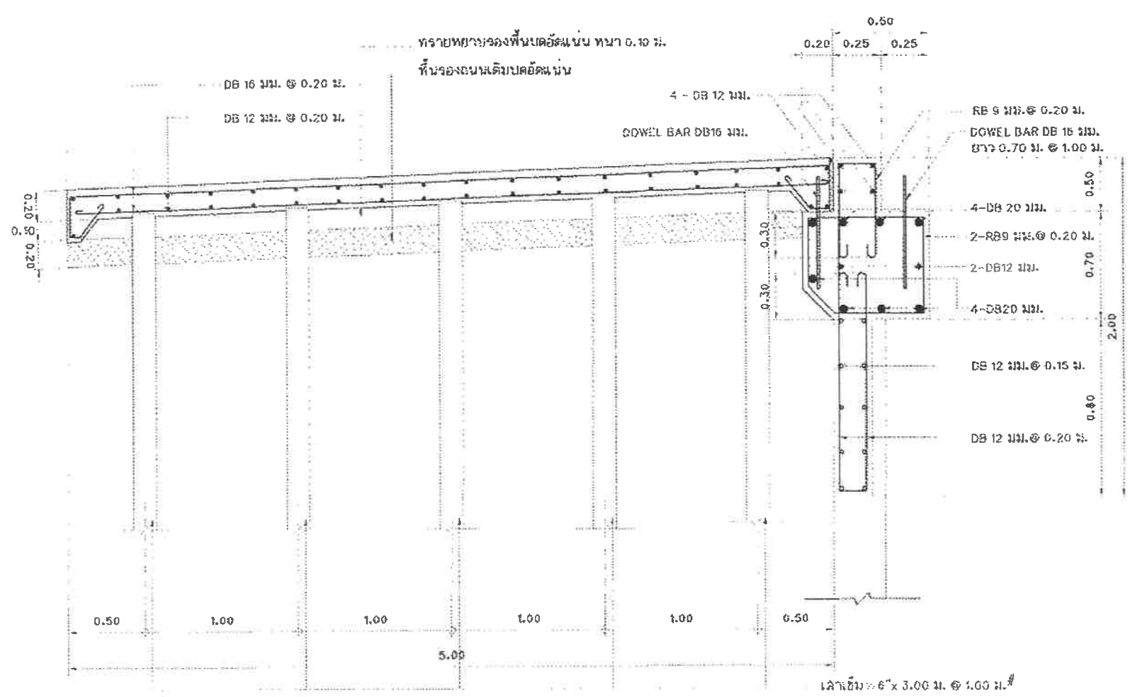
รูปตัดการเชื่อมสะพาน และพิวถนน คสล. (ฝั่งหมู่บ้านประชานีแคว้น 2 ระยะ 3) มาตรฐาน
