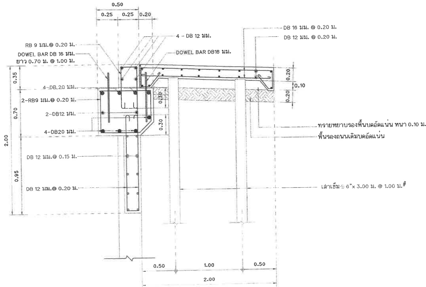
รูปตัดการเชื่อมสะพาน และผิวถนน คสล. มาตราส่วน 1 : 25
