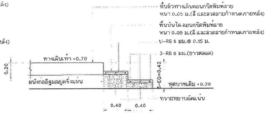
แบบขยายรูปตัดบ้นไค ST2 มาตราส่วน 1: 25
