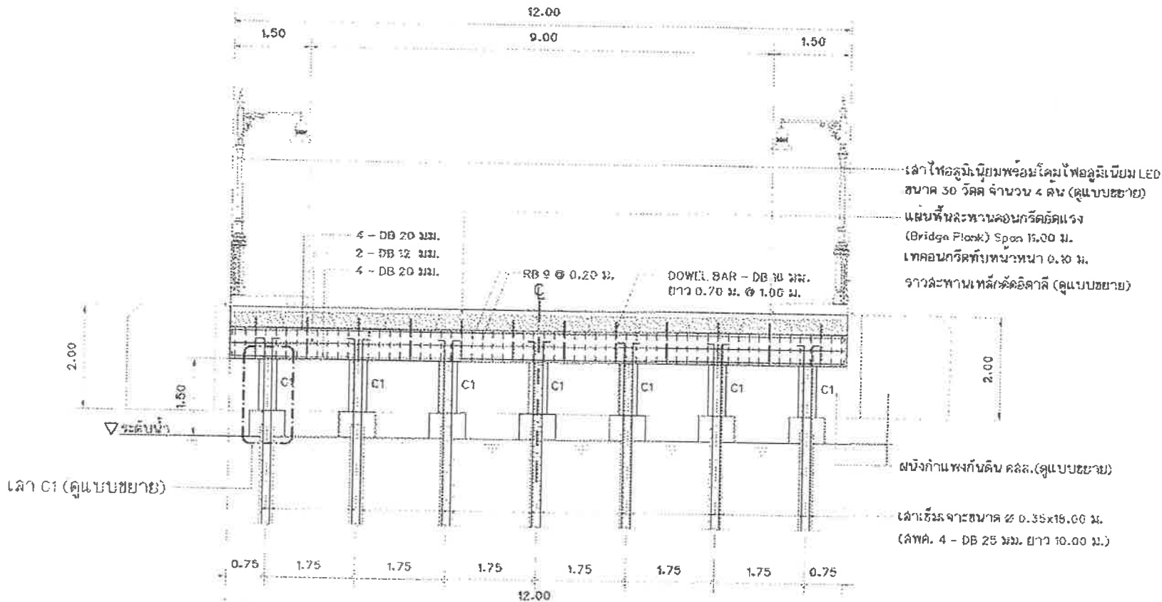
รูปตัดโครงสร้าง A - A (สะพานที่ 1) มาตรฐาน 1:75
