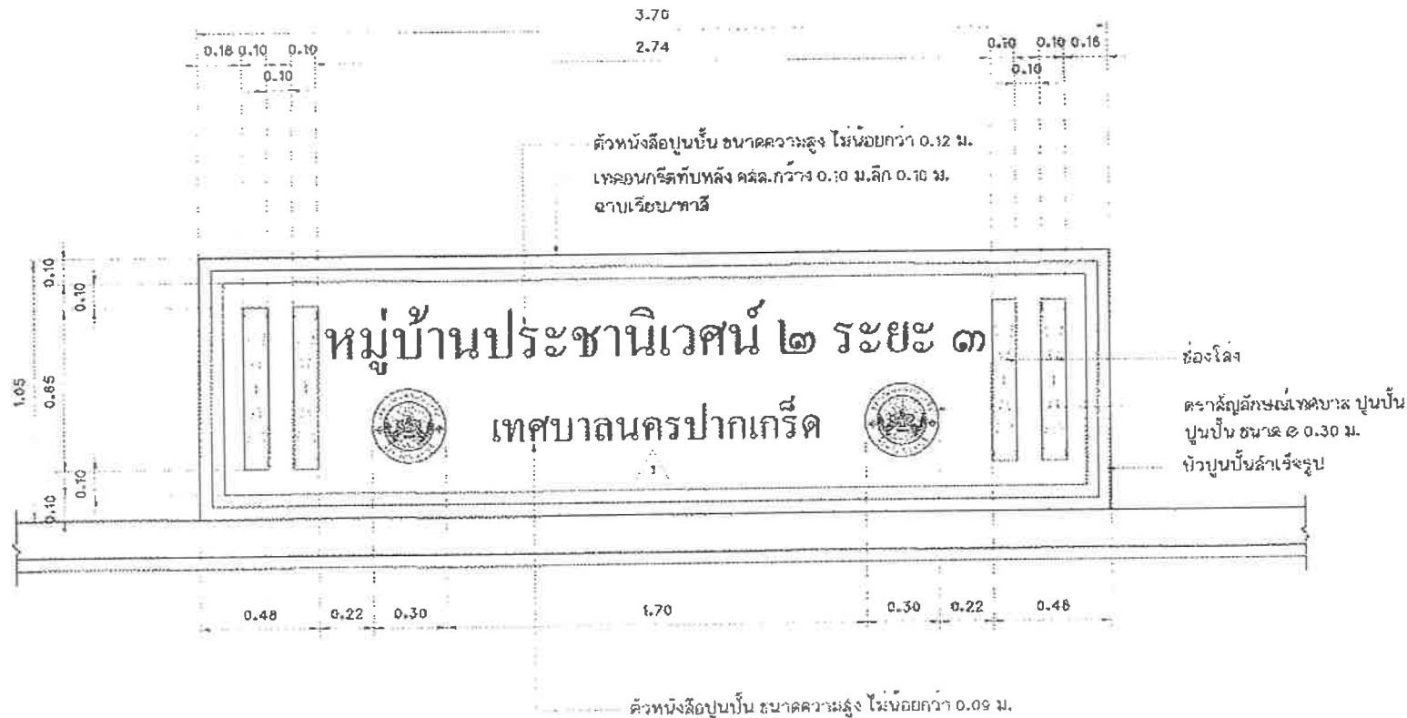
แบบขยายป้ายสะพาน คสล. มาตราส่วน 1:20
