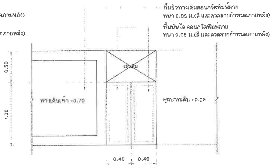
แบบขยายรูปตัดบ้นไค ST2 มาตราส่วน 1: 25
