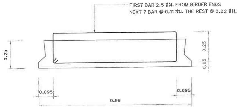
PLANK 8.00 ม. SPAN
