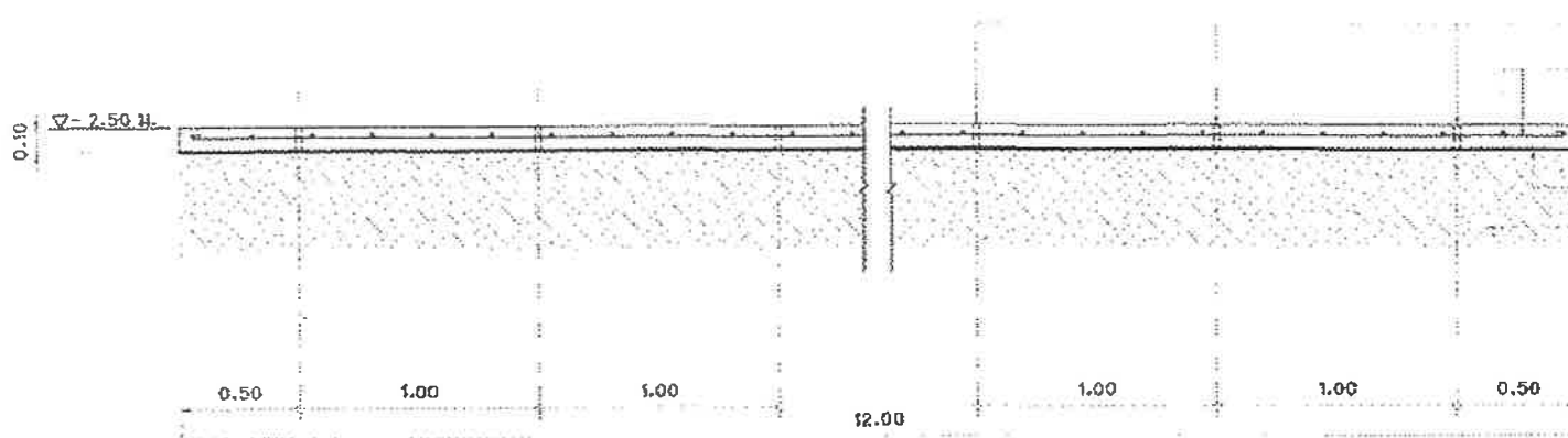
รูปตัดตามท่อคลอง (สะพานที่ ๑) มาตรฐาน ๑:๒๕
