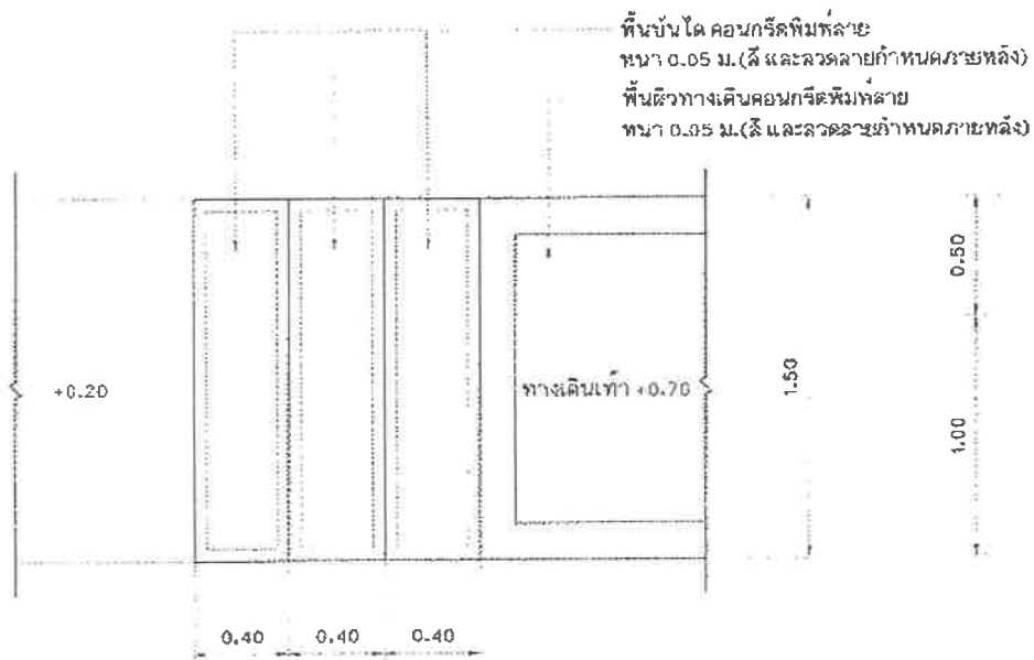
แบบขยายรูปตัดบ้นไค ST1 มาตราส่วน 1: 25
