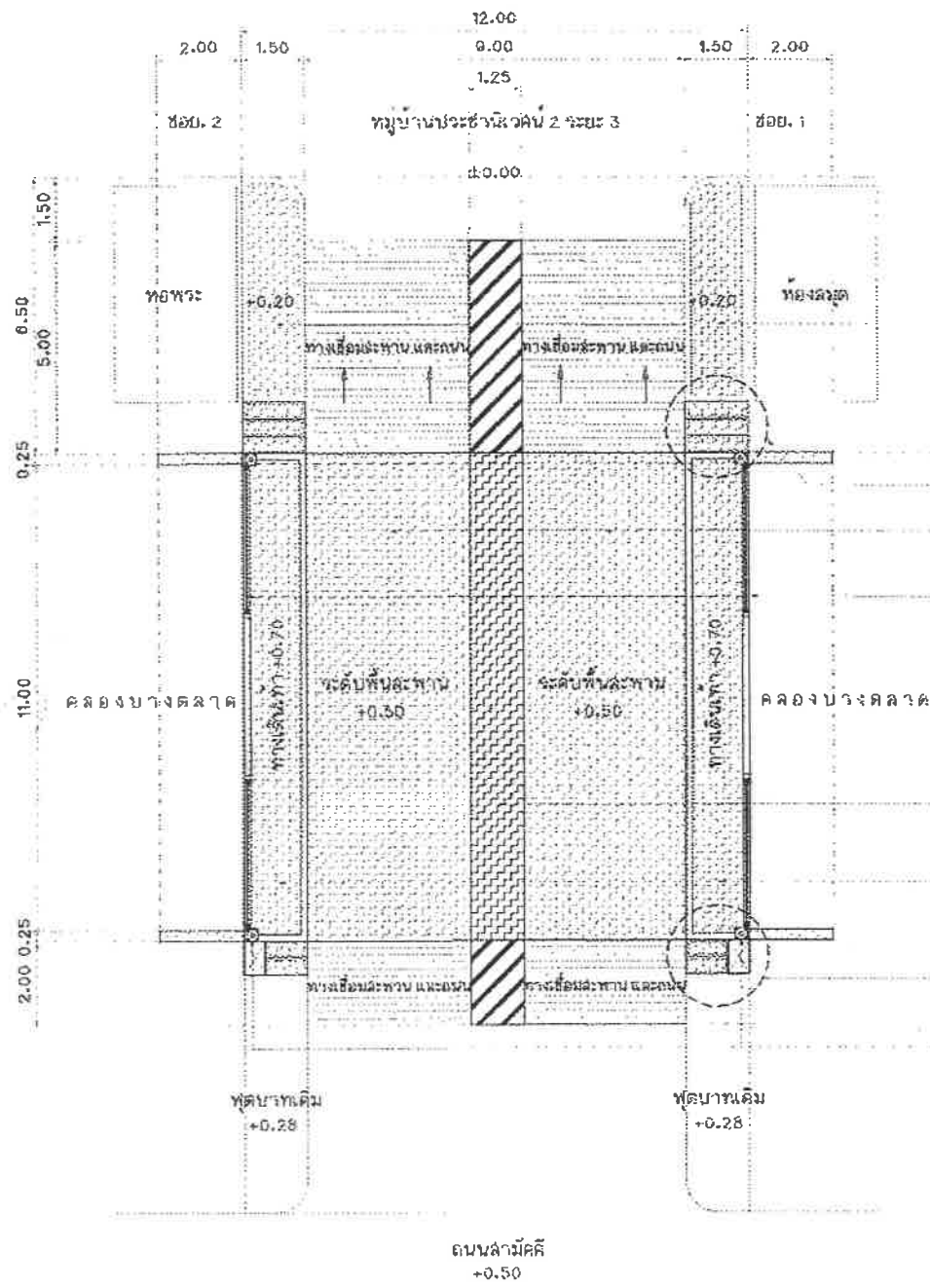
แปลนสะพาน คสล. (สะพานที่ 1) มาตราส่วน 1:125
