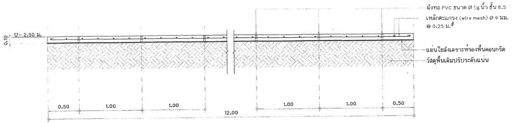
รูปตัดดาดท้องคลอง (สะพานที่ 2) มาตรฐาน 1:25
