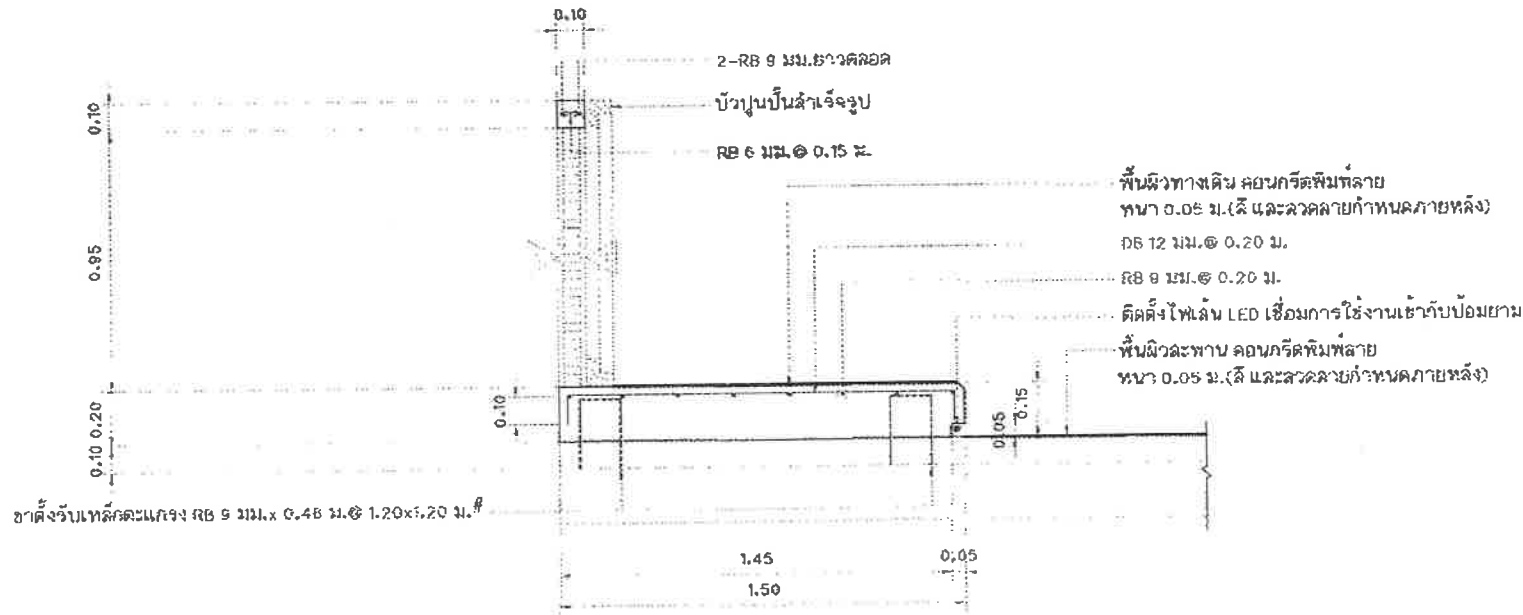
แบบขยายรูปตัดโครงสร้างป้ายสะพาน คลล์. พื้นทางเก่า มาตราส่วน 1: 20
