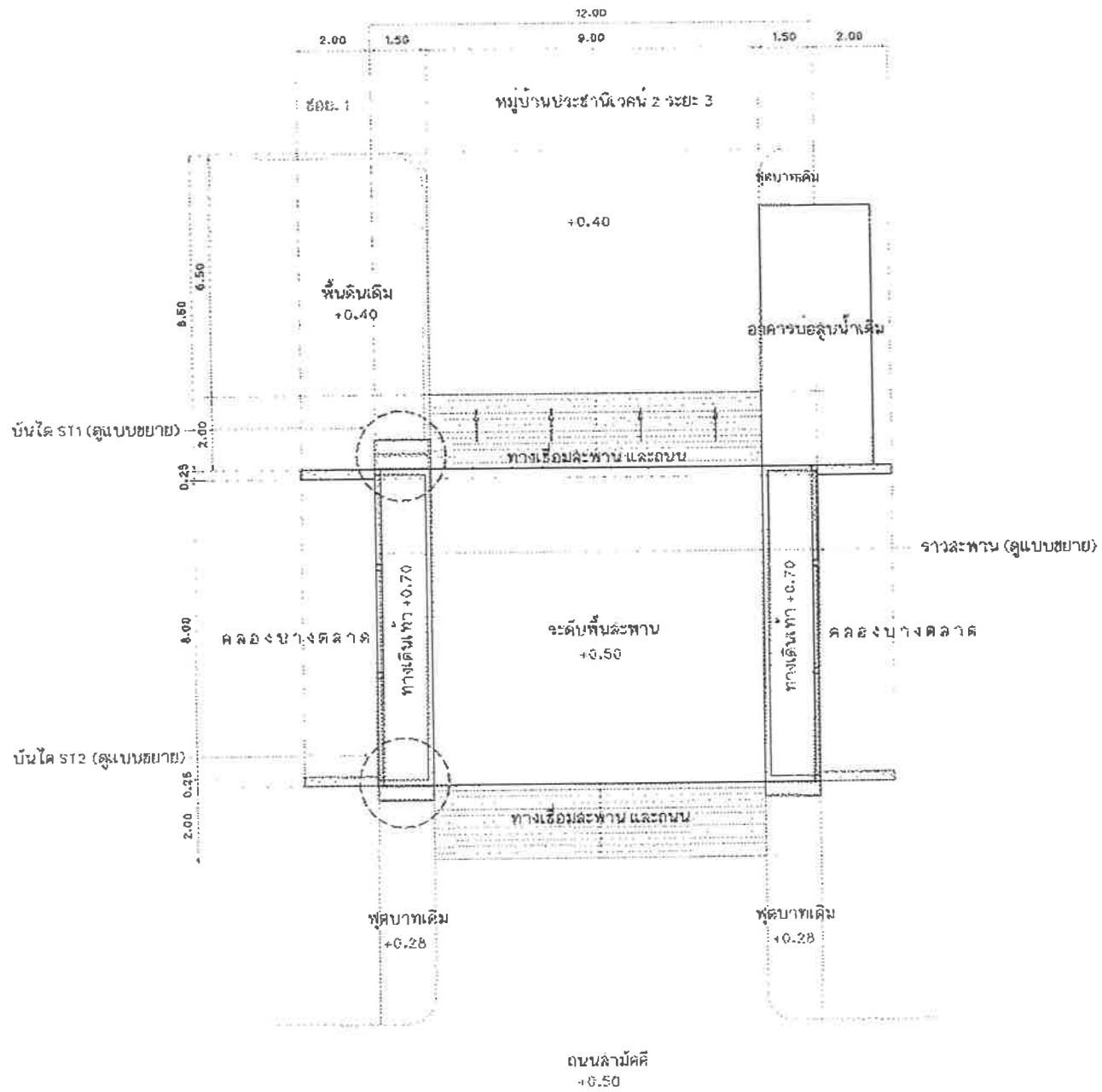
แปลนสะพาน คลล. (สะพานที่ 2) มาตรฐานจ.จ 1: 125
