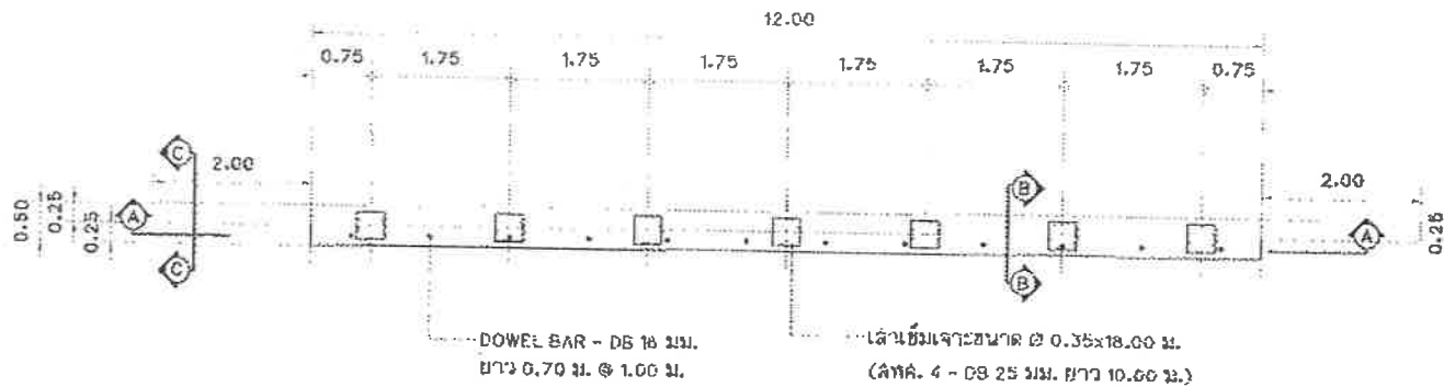
ขยายโครงสร้างสะพาน (สะพานที่ 1) มาตรฐาน 1:75
