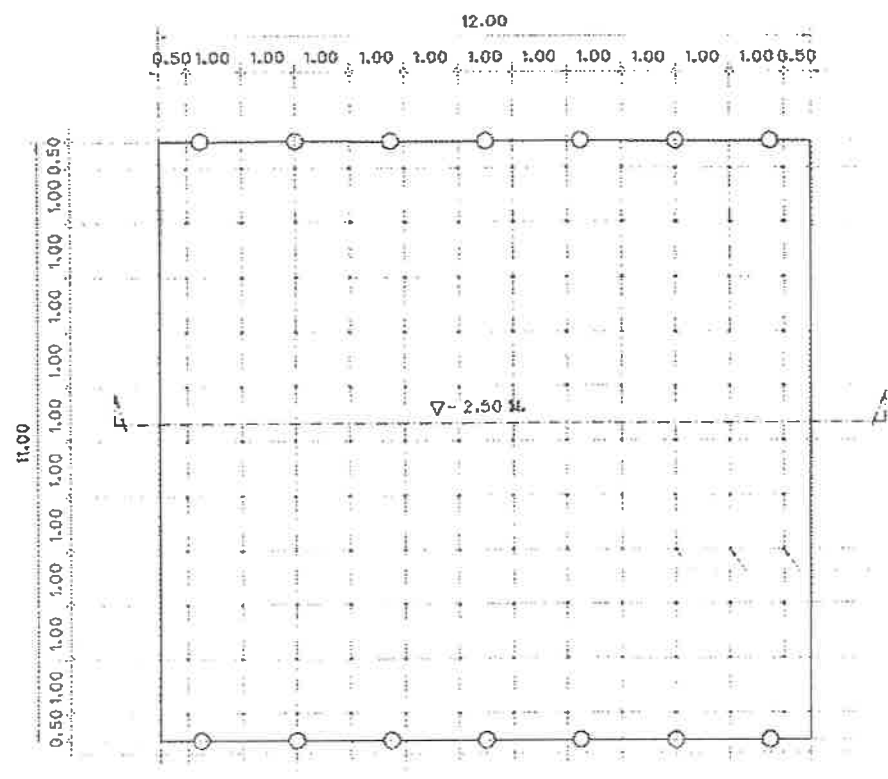
แปลนเสาเข็มตามท่อคลอง (สะพานที่ ๑) มาตรฐาน ๑:๑๐๐
