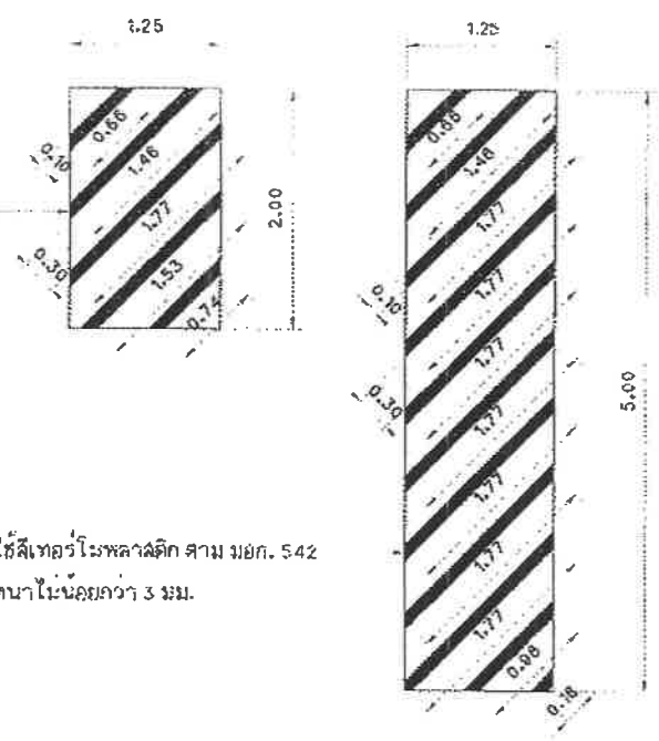
แบบขยายตีเส้นจราจรทางเชื่อมสะพาน และถนน คสล. มาตราส่วน 1:50
