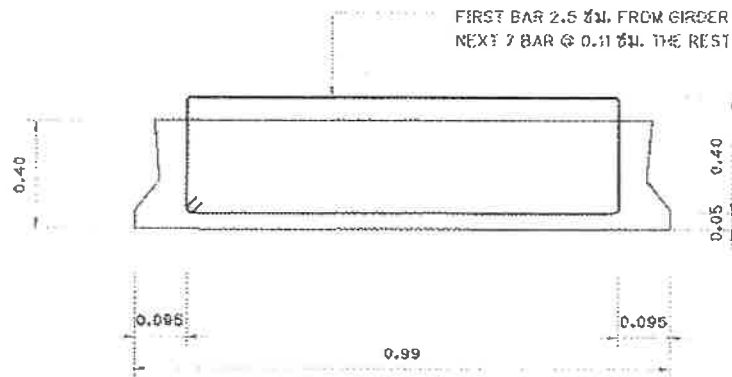
PLANK 11.00 M. SPAN
