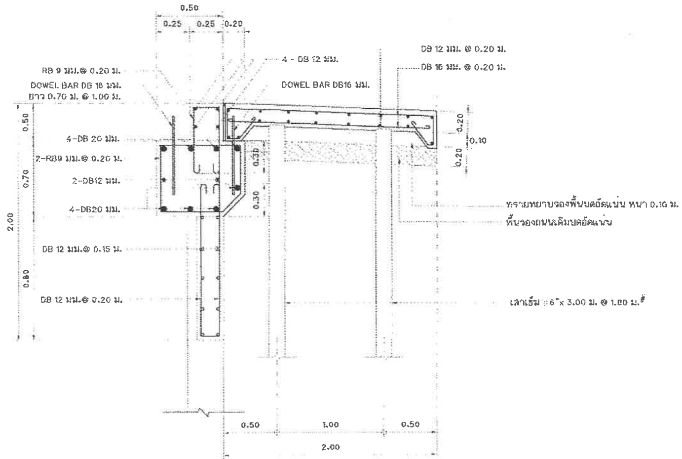
รูปตัดการเชื่อมสะพาน และฉีกรวม คสล. (ฝั่งถนนลำผักคี้)
