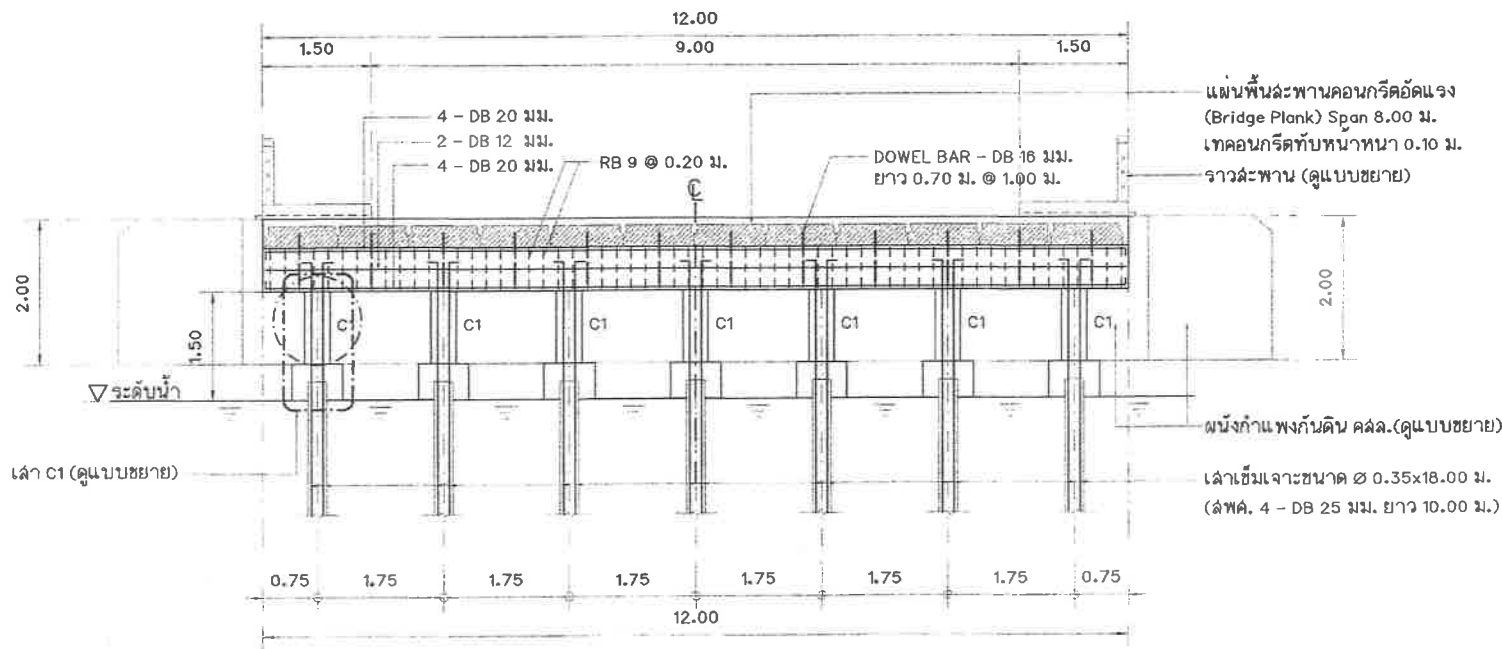
รูปตัดโครงสร้าง A - A (สะพานที่ 2) มาตราส่วน 1:75
