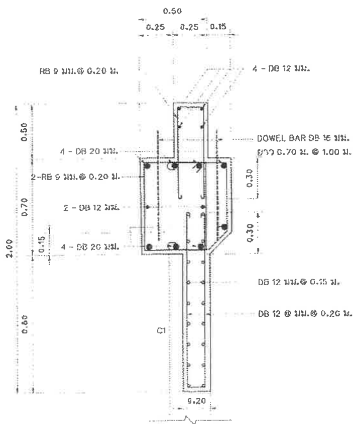
รูปตัดโครงสร้าง B - B (สะพานที่ 1) มาตราส่วน 1:20
