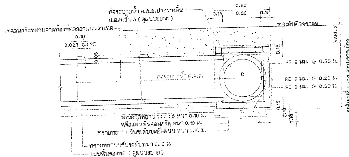
รูปตัดการเชื่อมต่อระบายน้ำของเดิม มาตราส่วน 1:25
