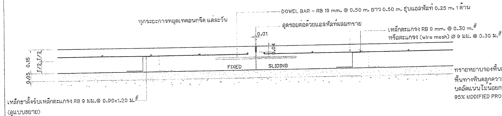
แบบขยาย CONSTRUCTION JOINT มาตราส่วน 1 : 10 ทุกระยะการหยุดเทคอนกรีต แต่ละวัน
