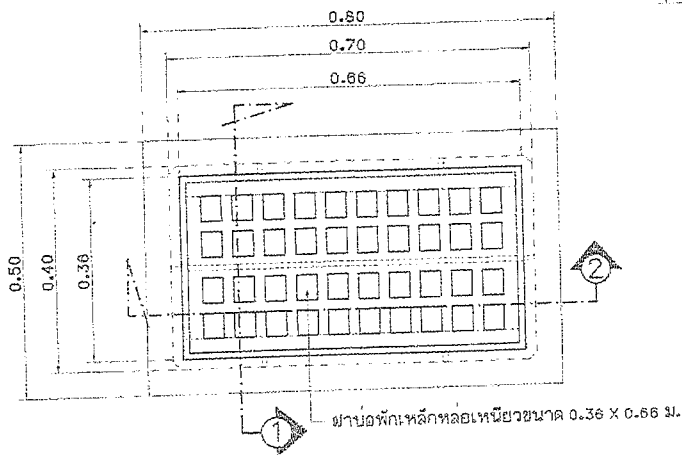
แบบขยายฝาบ่อพักรางวีเหล็กหล่อเหล็ย มาตราส่วน 1:10
