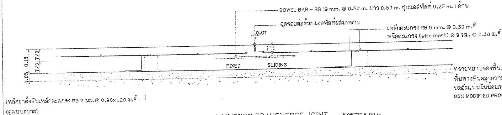
แบบขยาย TRANSVERSE JOINT มาตราส่วน 1 : 10 ทุกระยะ 6.00 ม.
