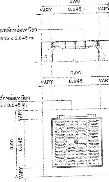
แบบขยายฝาบ่อพักเหล็กหล่อเหนียว 2 มาตราส่วน 1:20
