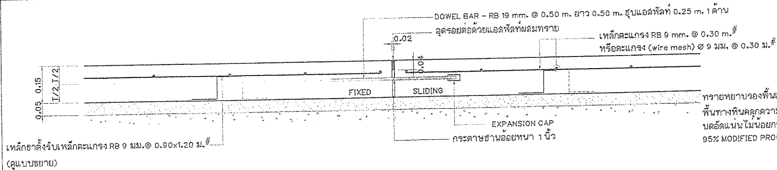
แบบขยาย EXPANSION JOINT มาตราส่วน 1 : 10 ทุกระยะ 30.00 ม.
