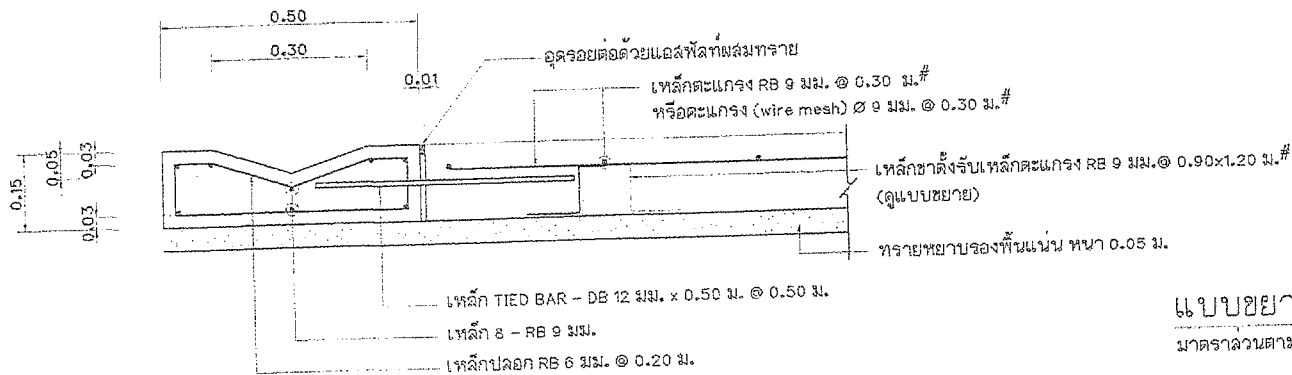
ขยายตัดขวางวิ คสล. มาตราส่วน 1 : 10
