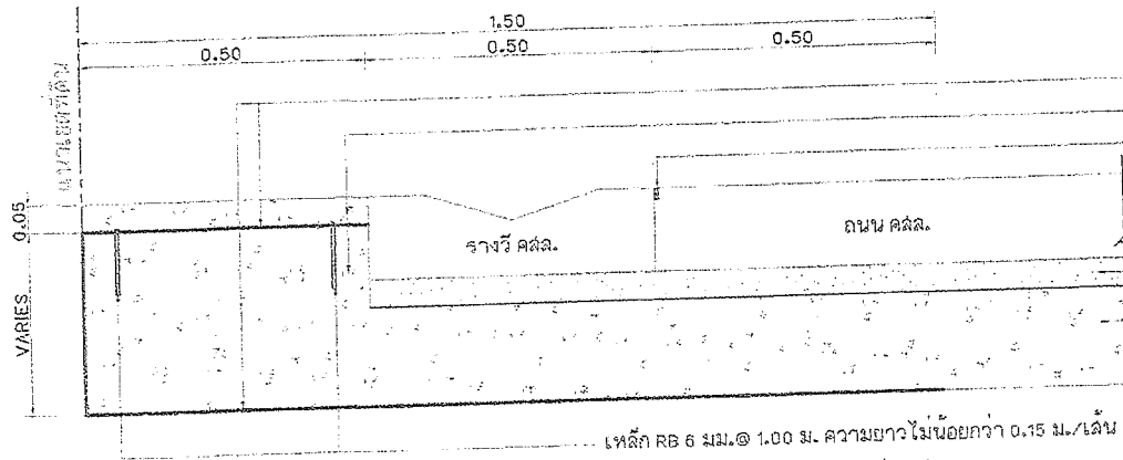
แบบขยายรูปตัดการติดตั้งแผ่นใยสังเคราะห์แผ่น มาตราส่วน 1 : 10
