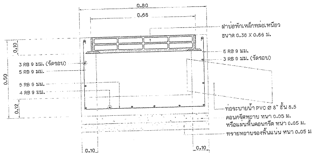
แบบขยายรูปตัด ② บ่อพักระบายน้ำ คลล. พร้อม ฝาบ่อพักรางวี มาตราส่วน 1:10
