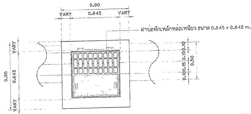
แบบขยายแปลนรางวี มาตราส่วน 1:20
