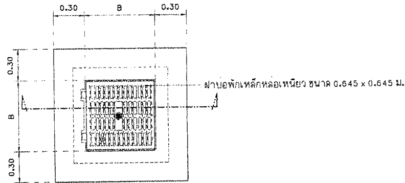
แปลนขยายบ่อพัก(หัวมุม)
