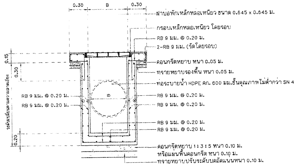
แบบขยายรูปตัดการเสริมเหล็ก บ่อพัก(หัวมุม)
