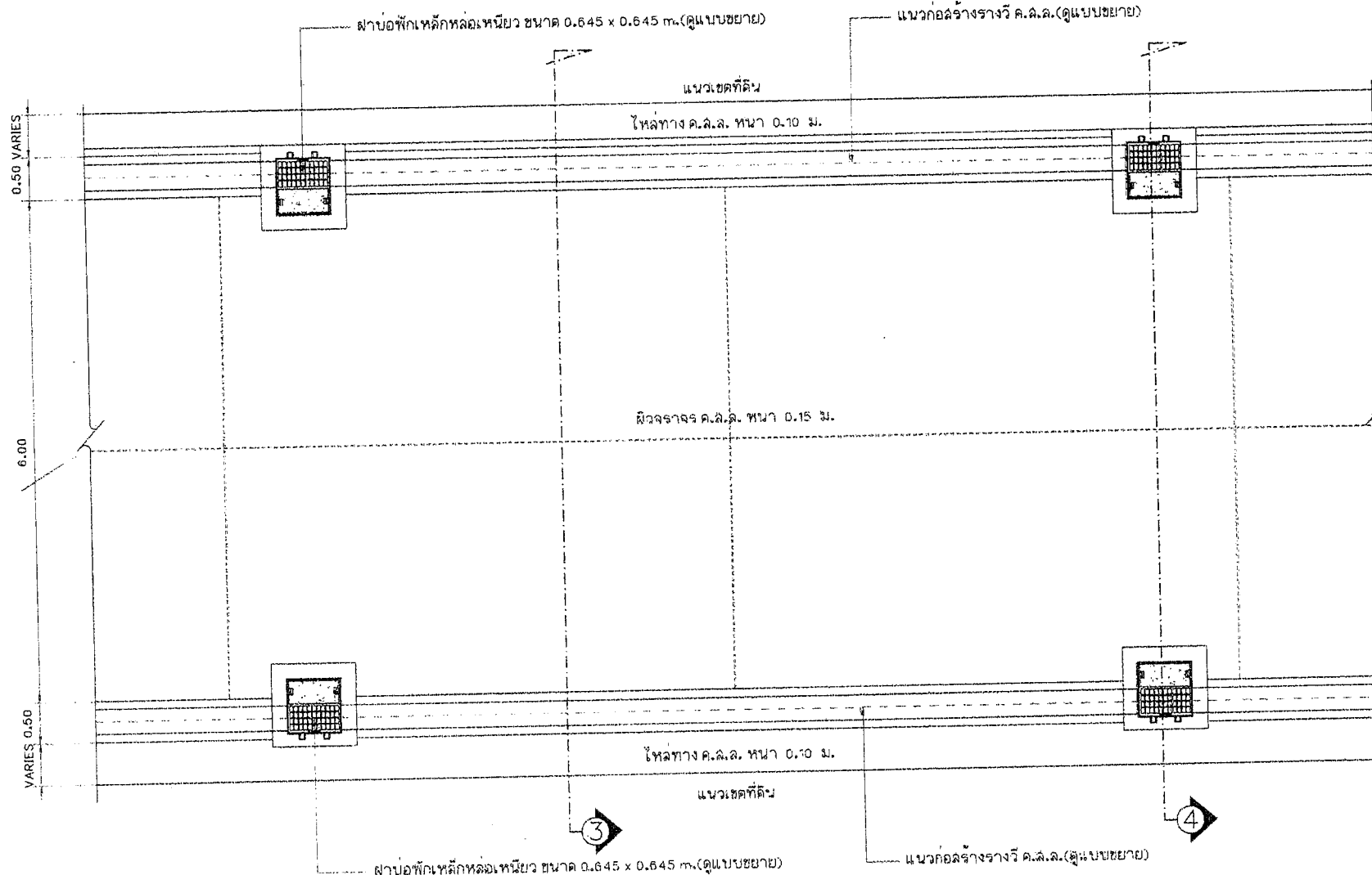
แปลนถนน และการวางบ่อพัก คสล. ช่วง 6.00 เมตร มาตราส่วน 1 : 50
