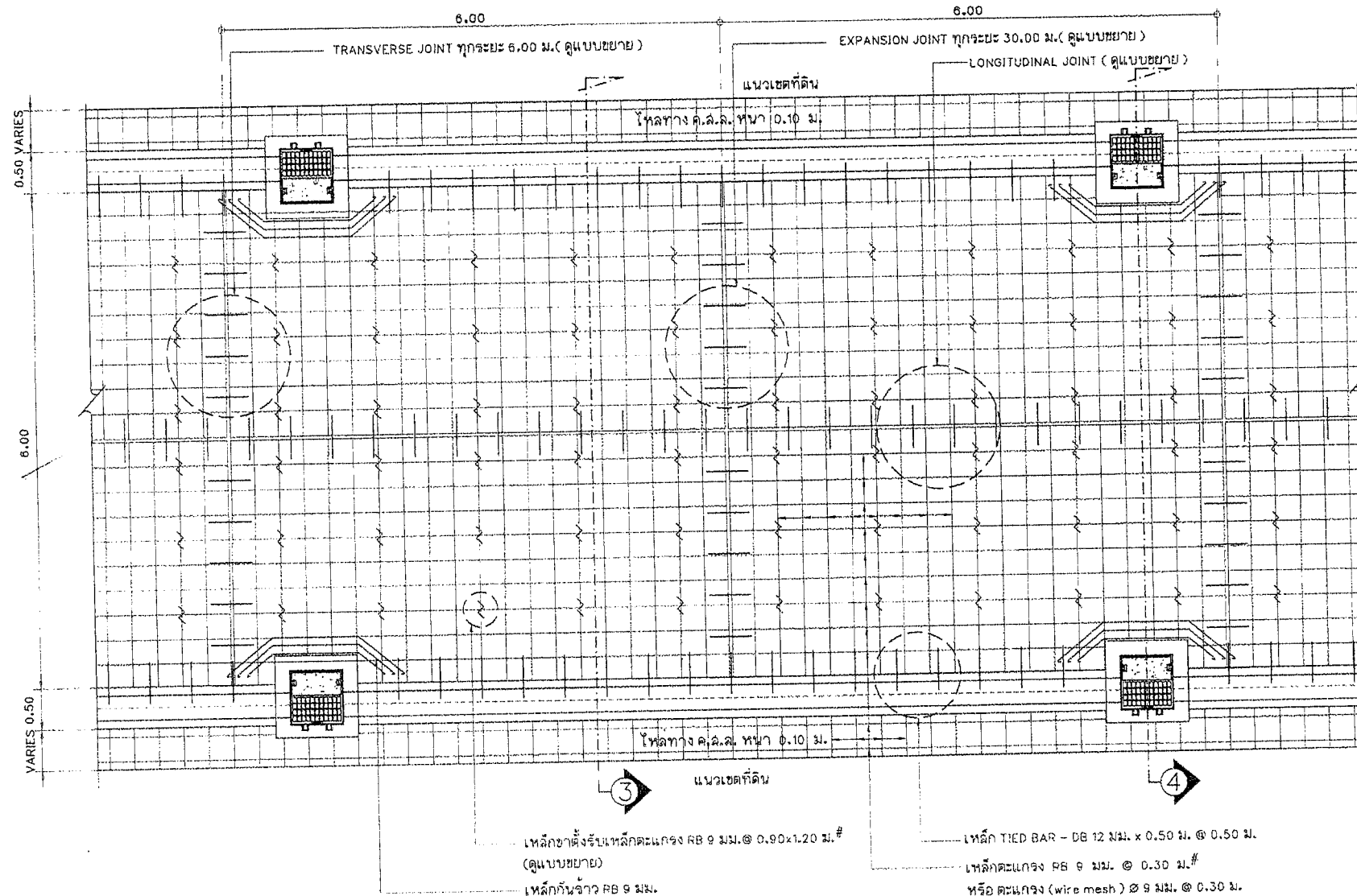
แปลนการวางเหล็กดัดแครงและรอยต่อนน คสล. ช่วง 6.00 เมตร
