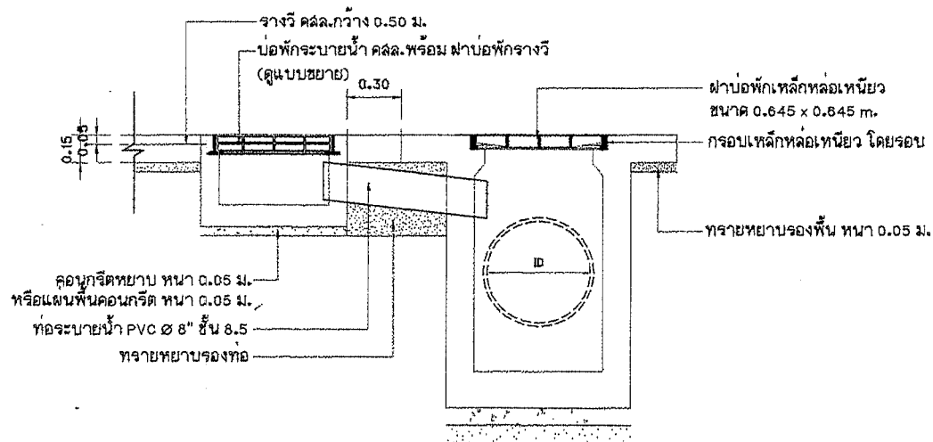
แบบขยายรูปตัดการเชื่อมต่อท่อ บ่อพัก(หัวมุม) (จำนวน 4 บ่อ)
