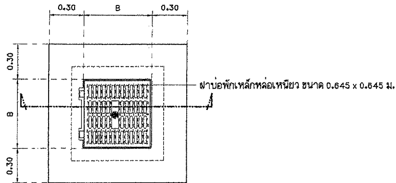
แปลนขยายบ่อพัก(หัวมุม) มาตราส่วน 1:25
