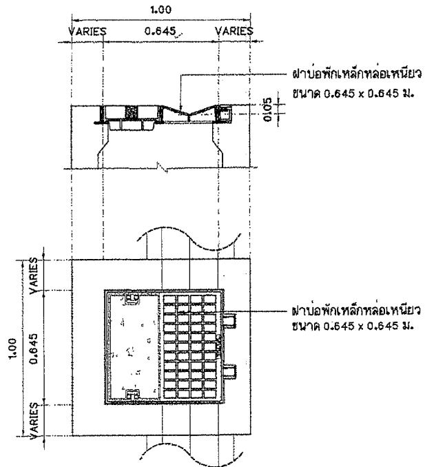
แบบขยายฝาบ่อพักเหล็กหล่อเหนียว 1 มาตราส่วน 1:20
