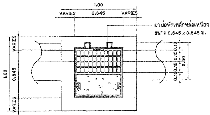
แบบขยายฝาบ่อพักเหล็กหล่อเหนียว 1 มาตราส่วน 1:20
