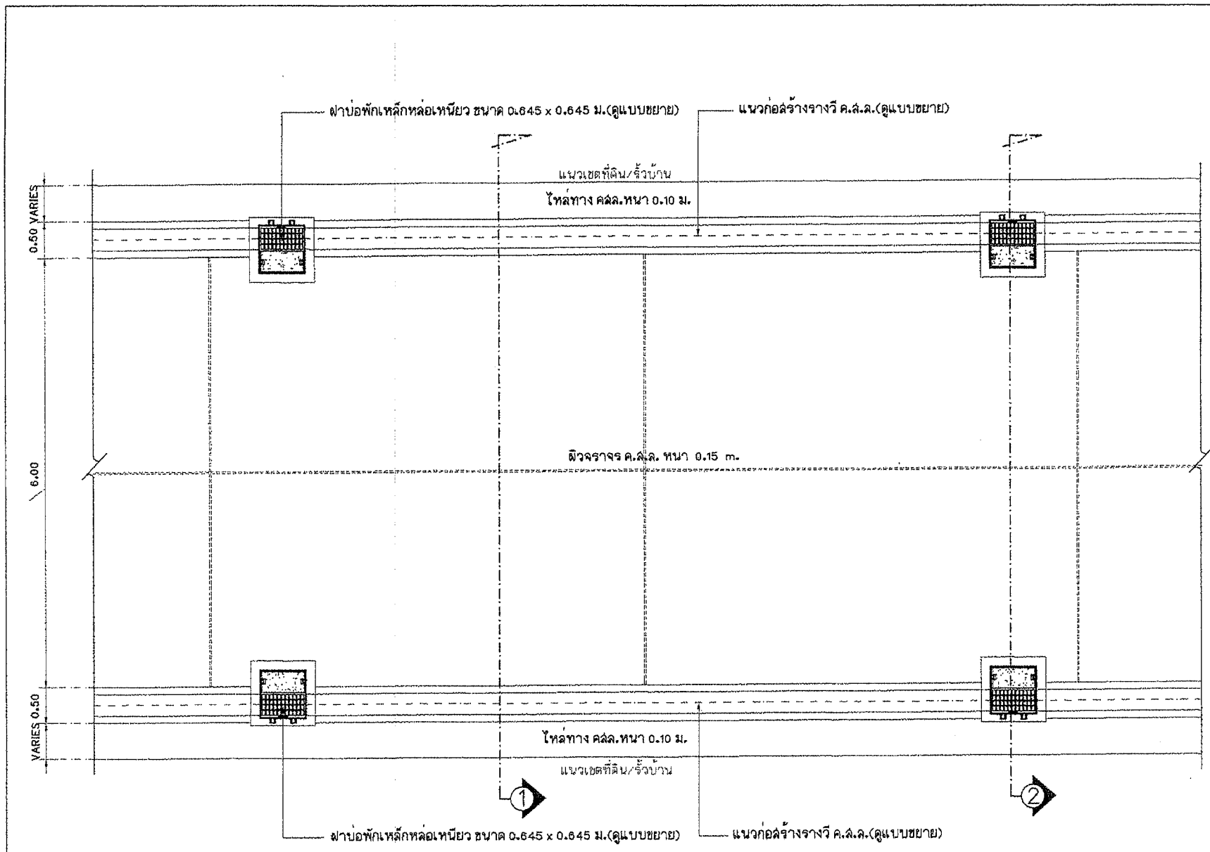
แผนถนน และการวางบ่อพัก ค.ล.ล. ช่วง 6.00 เมตร มาตราส่วน 1 : 50
