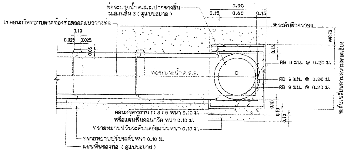
รูปตัดการเชื่อมต่อในกรณีเชื่อมกับท่อระบายน้ำของเดิม มาตราส่วน 1:20
