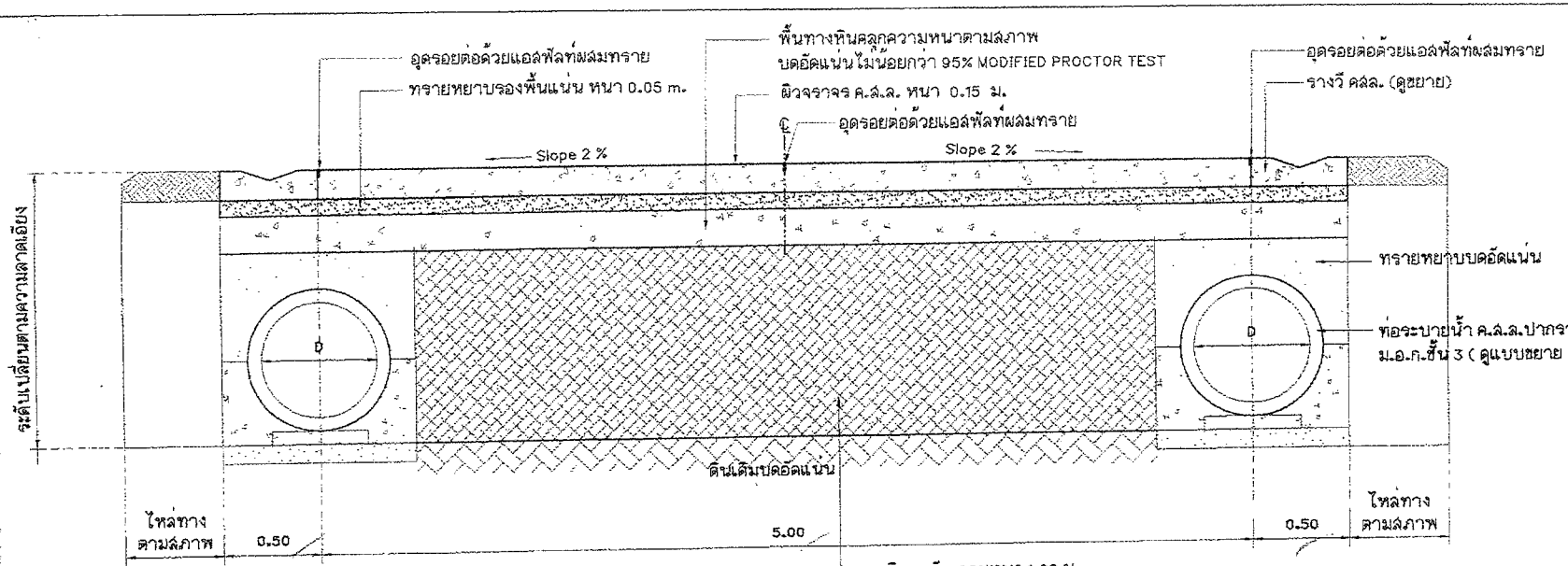
แบบขยายรูปตัด 1 มาตราส่วน 1:20
