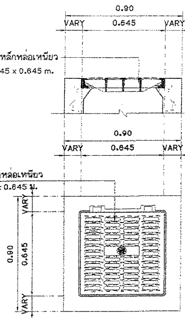
แบบขยายฝาบ่อพักเหล็กหล่อเหนียว 2 มาตราส่วน 1:20
