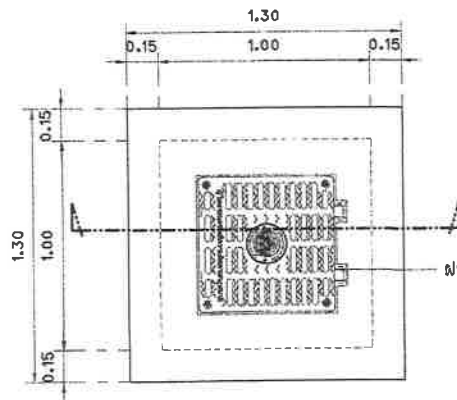
แบบขยายบ่อพักหัวมุม มาตราส่วน 1:25
