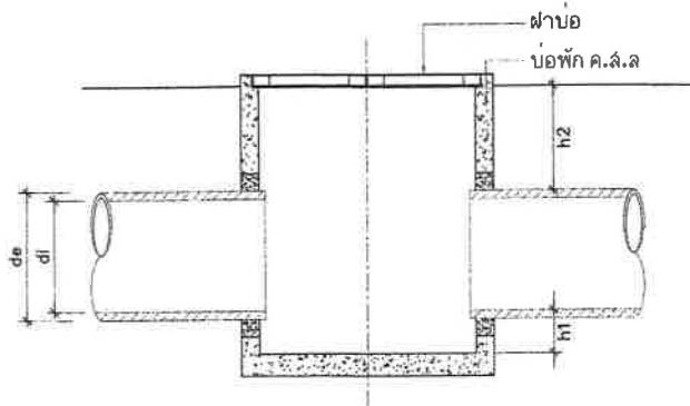
การประลันท่อ HDPE เข้าบ่อ ค.ส.ล. มาตรฐานตามกำหนด
