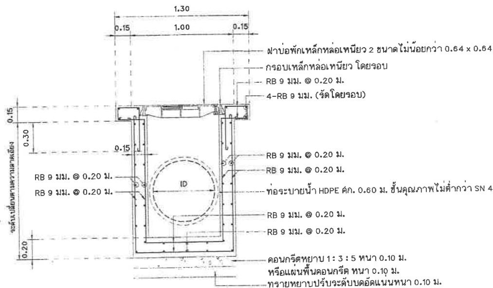
แบบขยายรูปตัดการเสริมเหล็กบ่อพักหัวมุม มาตราส่วน 1:25
