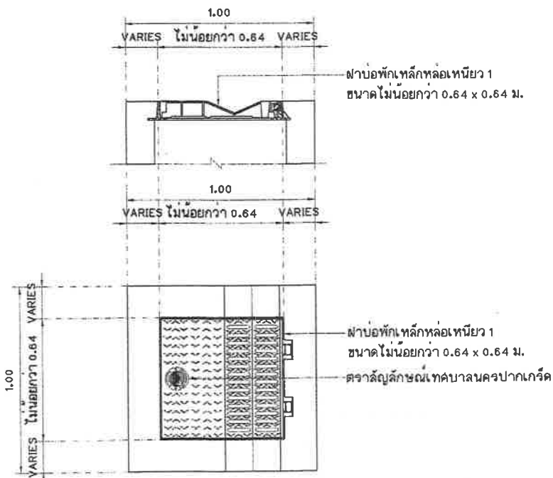
แบบขยายฟาบ่อพักเหล็กหล่อเหนียว 1 มาตราส่วน 1:20
