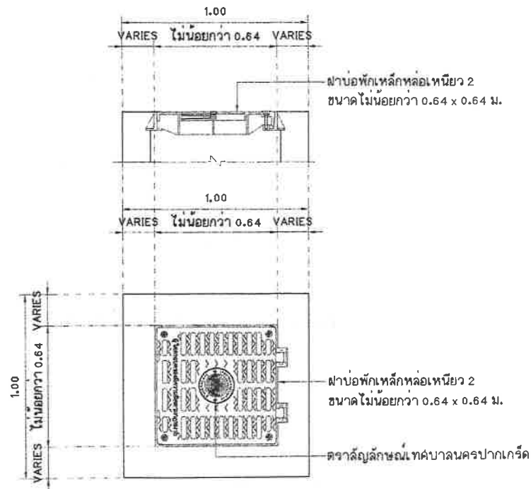
แบบขยายฟาบ่อพักเหล็กหล่อเหนียว 2 มาตราส่วน 1:20 (ฟาบ่อพัก และกรอบเป็นชนิดกันเลียงโดยเฉพาะ)
